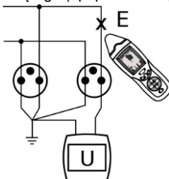
Rys. 8 Schemat trybu napięciowego.
