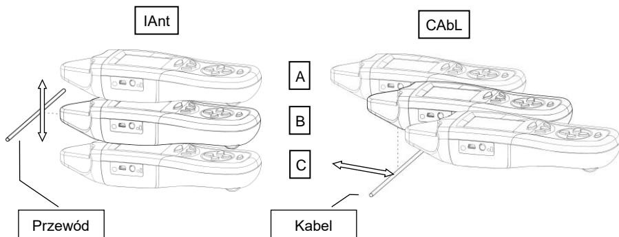
Rys. 20 Lokalizacja przewodu / kabla położonego prostopadle do osi symetrii odbiornika.
