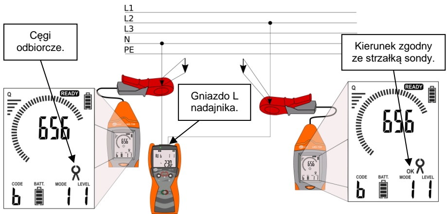
Rys. 40 Cęgi odbiorcze – wymuszenie prądowe w zlokalizowanym obwodzie.
